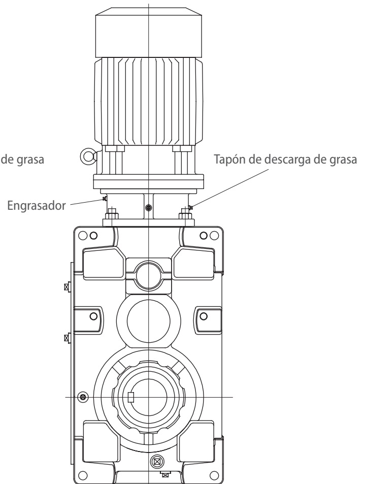
Fig. 4 - Unidad de accionamiento, montaje perpendicular
