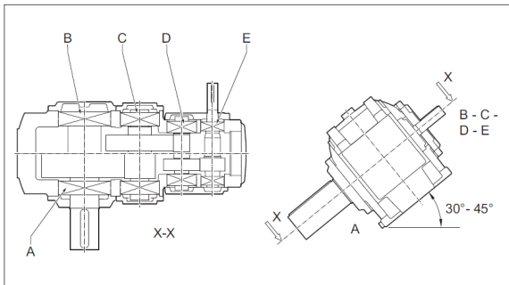
A: Punto de lubricación en el nivel inferior
